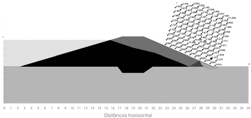
Figura 1 - Análise de estabilidade do talude de jusante da configuração hipotética 1 para a condição de reservatório cheio.
