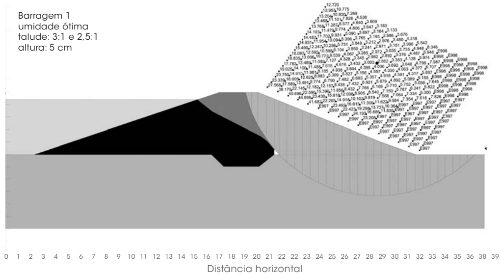
Figura 2 - Análise de estabilidade do talude de jusante da configuração hipotética 2 para a condição de reservatório cheio. Fonte: Elaboração própria.
