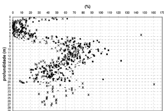
Figura 5: Variação do coeficiente de atrito f_r (%) com a profundidade
