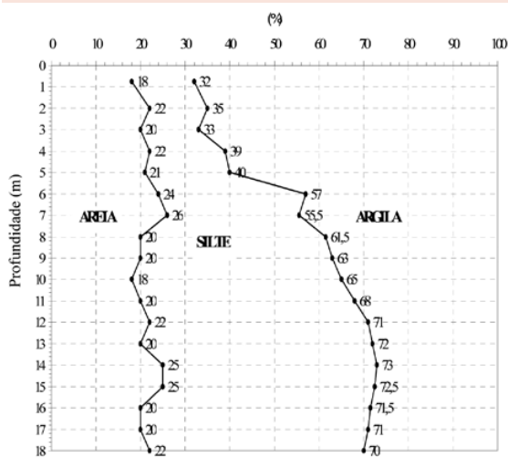
Figura 2: Variabilidade granulométrica do subsolo do Campo Experimental
