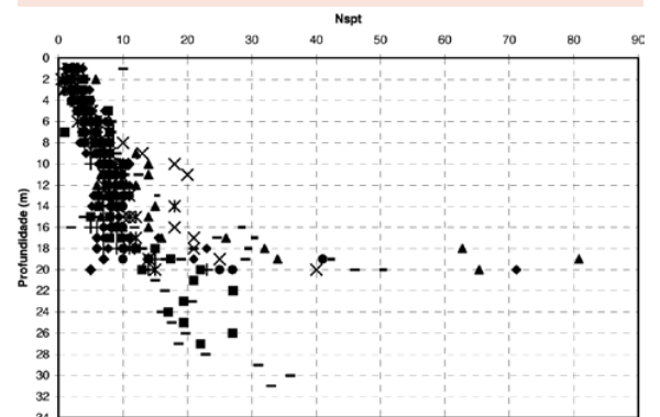
Figura 3: Variação do N_{spt} com a profundidade
