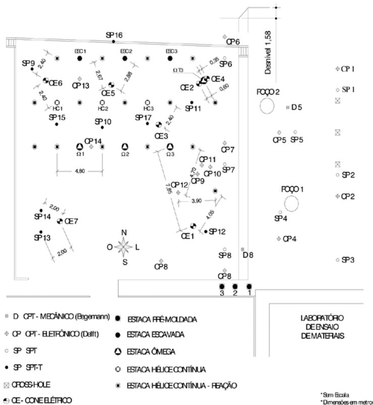
Figura 1: Vista superior do Campo Experimental
