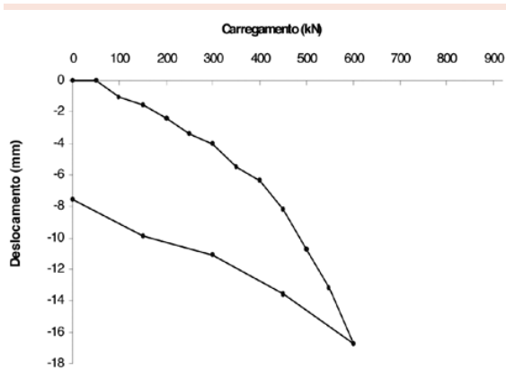
Figura 8: Curva carga recalque. Estaca HC-3.
