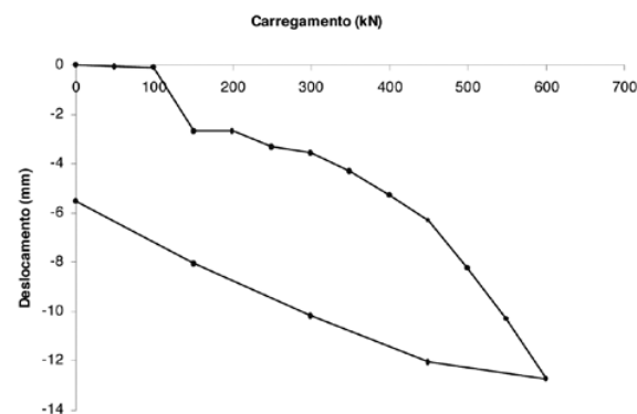
Figura 7: Curva carga recalque. Estaca HC-2
