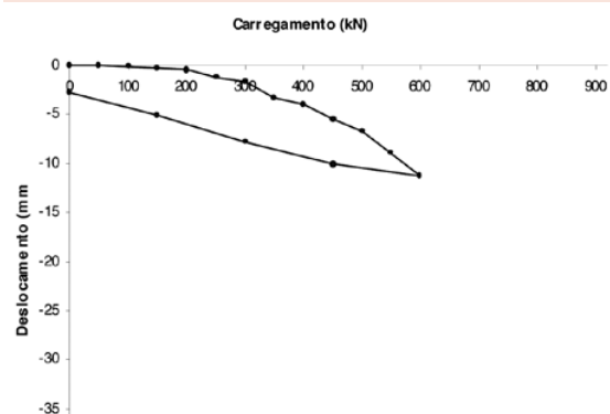
Figura 6: Curva carga recalque. Estaca HC-1
