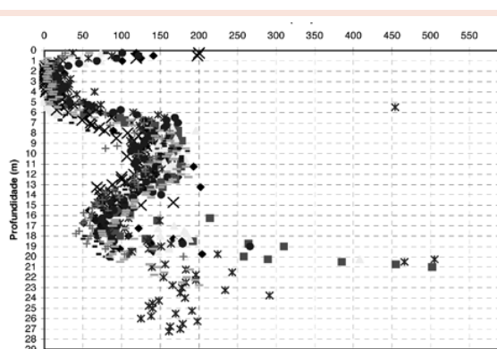
Figura 4: Variação do f_s (kPa) com a profundidade
